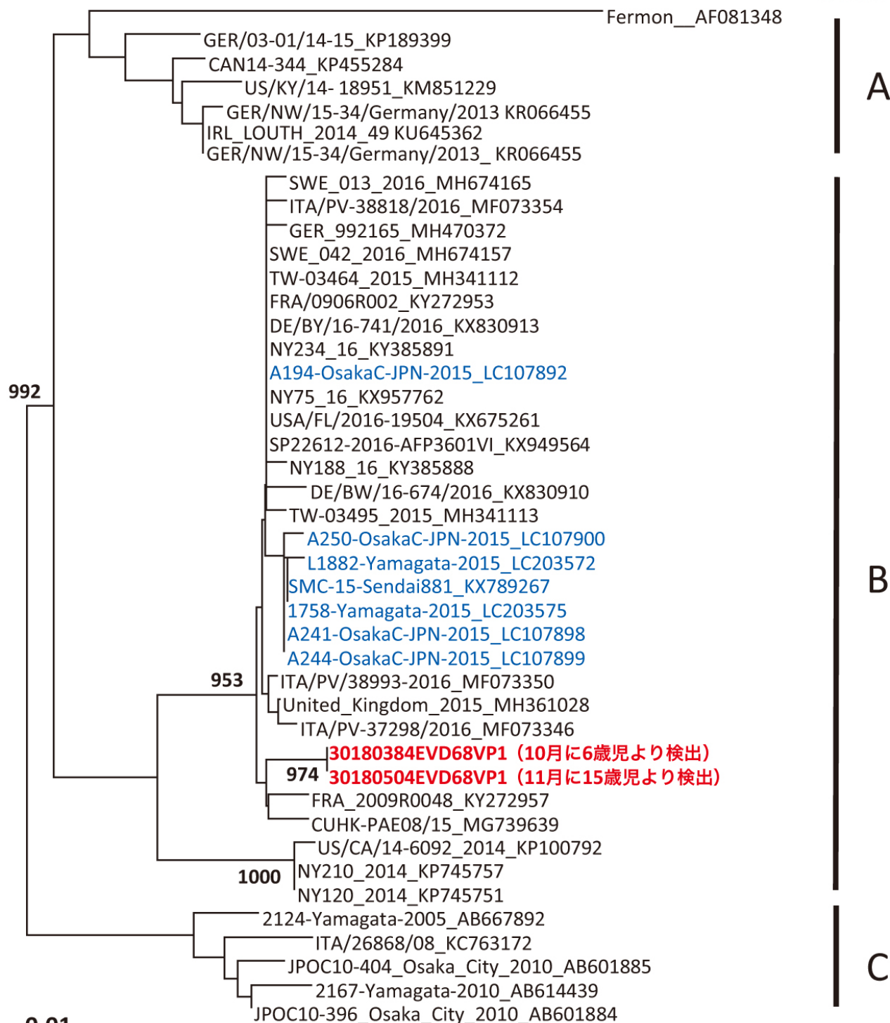
図2. 近隣結合法による近縁系統樹解析：VP1領域の一部 (369塩基) (bootstrap value > 950)
