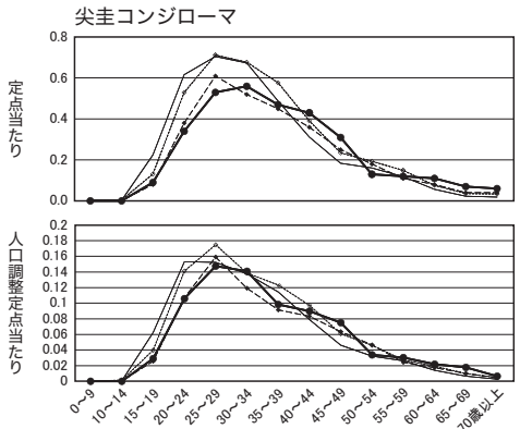
図1. 定点把握4疾患の定点当たり報告数および人口調整定点当たり報告数、2003～2012年
