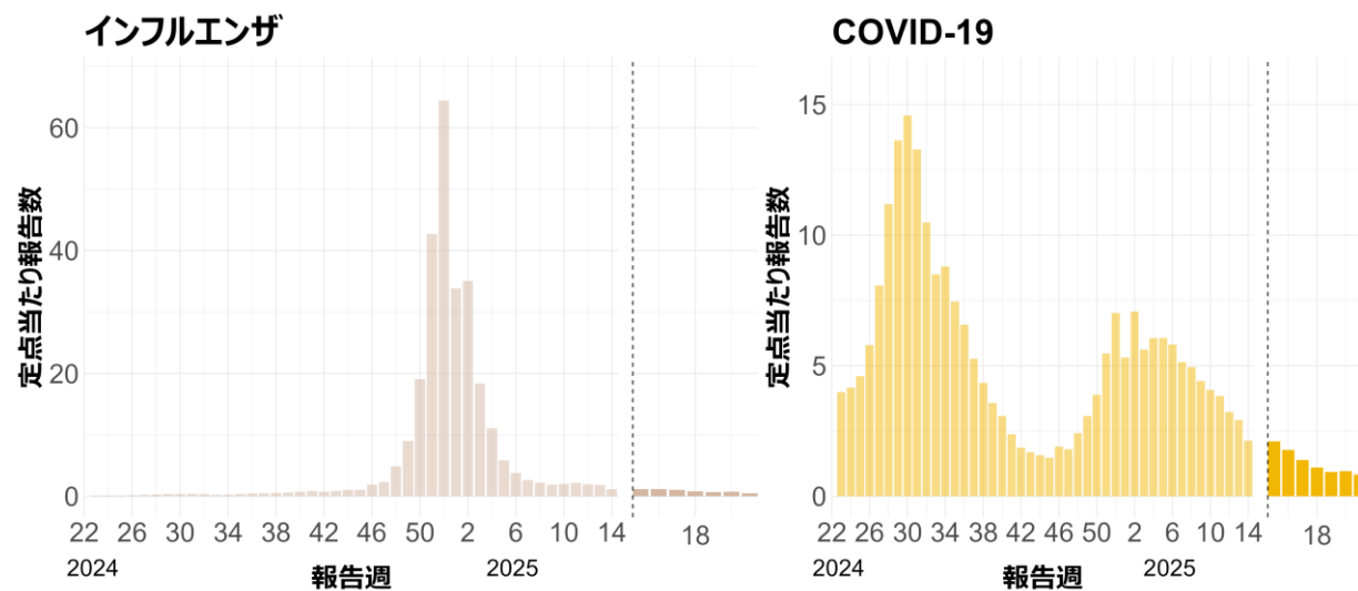
図 1B: 週ごとの感染症別の定点当たり報告数
