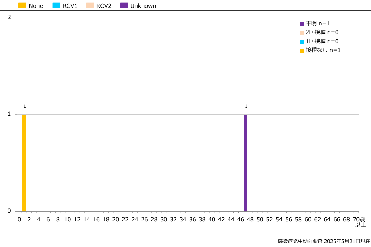
5-1. 年齢群別接種歴別風しん累積報告数 (男性) 2025年 第1~20週 (n=2) Cumulative rubella cases (male) by age and vaccinated status, week 1-20, 2025 (as of May 21, 2025)
